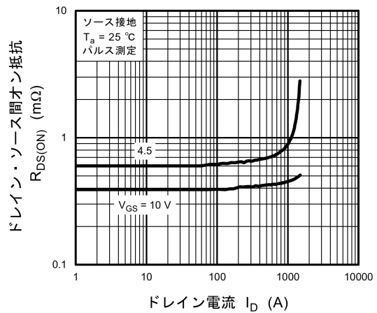
図 8.4 R_{DS(ON)} - I_D
