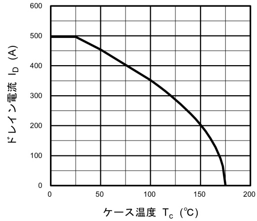
図 8.15 I_D - T_c
