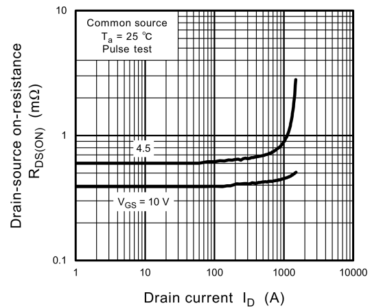
Fig. 8.4 R_{DS(ON)} - I_D
