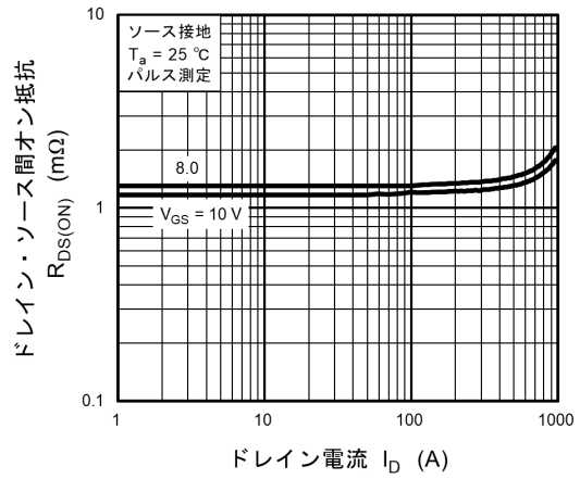
図 8.4 R_{DS(ON)} - I_D
