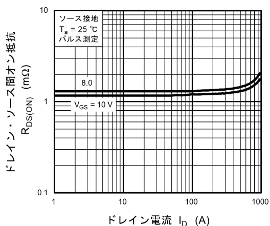
図 8.4 R_{DS(ON)} - I_D
