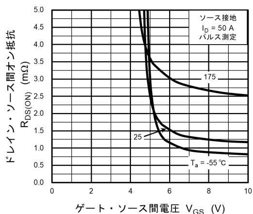
図 8.3 R_{DS(ON)} - V_{GS}
