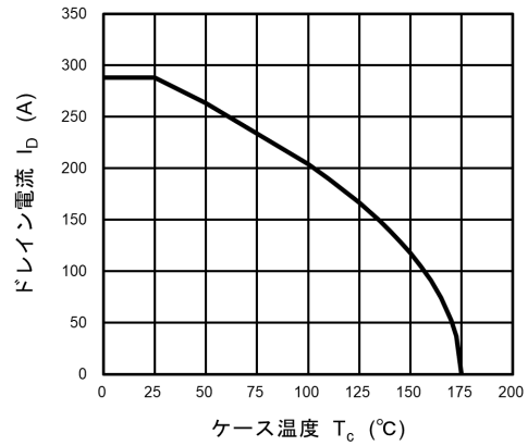
図 8.15 I_D - T_c
