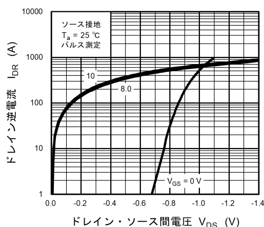
図 8.5 I_{DR} - V_{DS}
