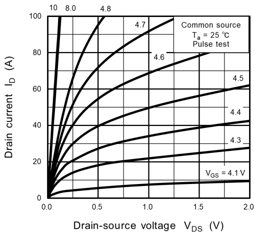
Fig. 8.1 I_D - V_{DS}
