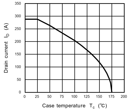
Fig. 8.15 I_D - T_c
