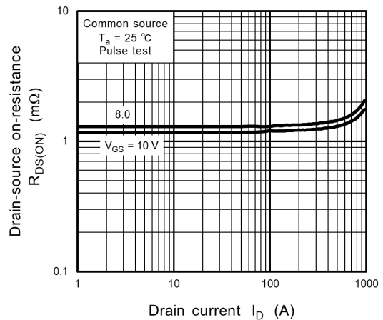
Fig. 8.4 R_{DS(ON)} - I_D
