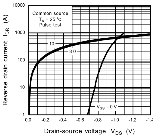
Fig. 8.5 I_{DR} - V_{DS}
