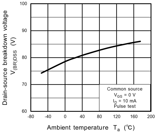
Fig. 8.7 V_{(BR)DSS} - T_a
