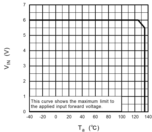
Fig. 12.1 V_{IN} - T_a
