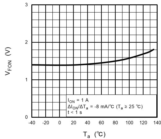
Fig. 12.6 V_{FON} - T_a
