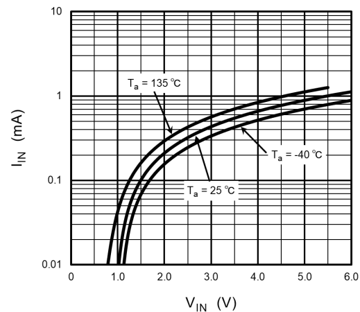
Fig. 12.2 I_{IN} - V_{IN}
