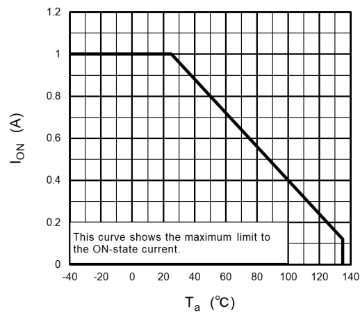
Fig. 12.3 I_{ON} - T_a
