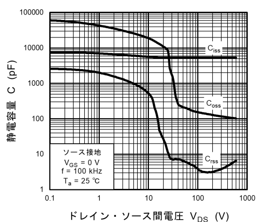
図 8.9 C - V_{DS}
