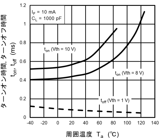
図 11.8 t_{on}, t_{off} - T_a
