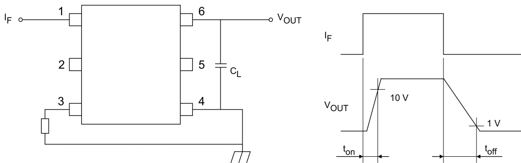
図 10.1 スイッチング時間測定回路, 波形
