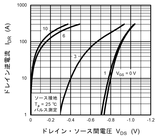
図 8.10 I_{DR} - V_{DS}
