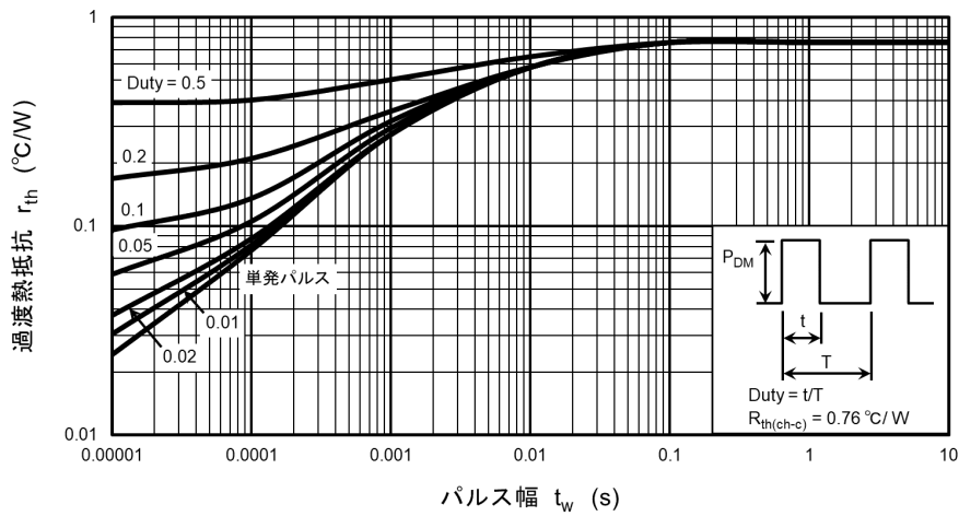
図 8.15 Z_{th(ch-c)} - t_w (最大値 (保証値))
