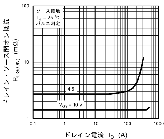
図 8.4 R_{DS(ON)} - I_D
