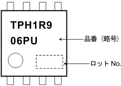
図 7.1 現品表示
