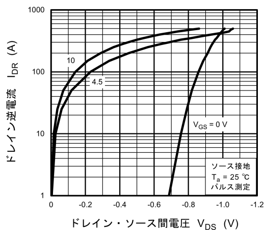
図 8.5 I_{DR} - V_{DS}
