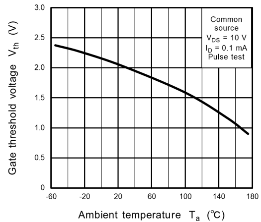
Fig. 8.6 V_{th} - T_a
