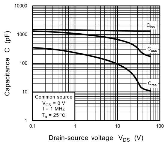
Fig. 8.7 C - V_{DS}
