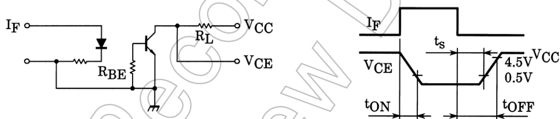
図 1: スwitchング時間測定回路
