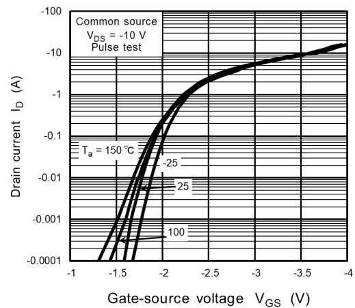
Fig. 9.2 I_D - V_{GS}
