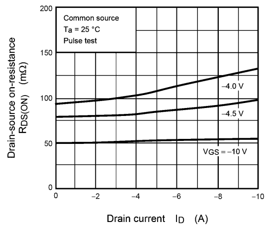
Fig. 9.4 R_{DS(ON)} - I_D
