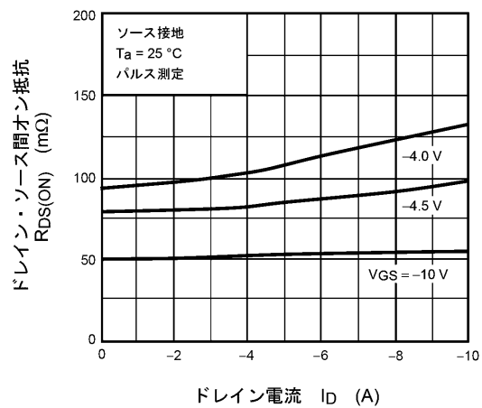
図 9.4 R_{DS(ON)} - I_D
