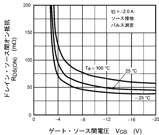
図 9.3 R_{DS(ON)} - V_{GS}
