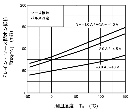
図 9.5 R_{DS(ON)} - T_a
