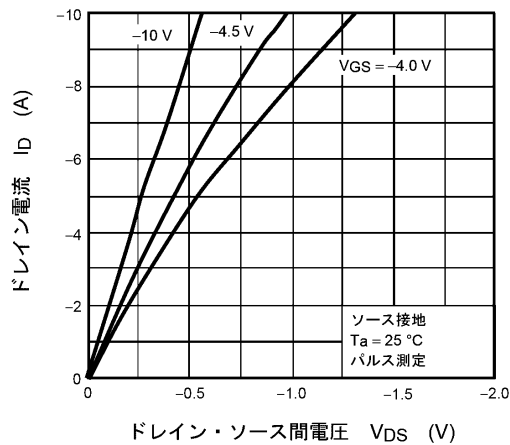
図 9.1 I_D - V_{DS}
