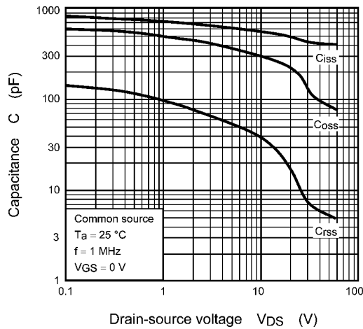
Fig. 9.7 C - V_{DS}
