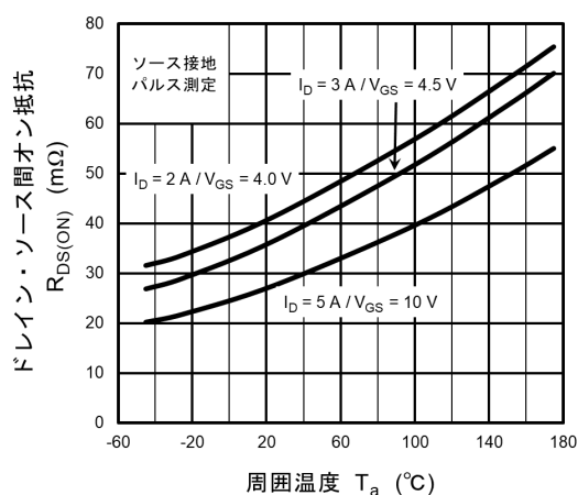
図 9.5 R_{DS(ON)} - T_a
