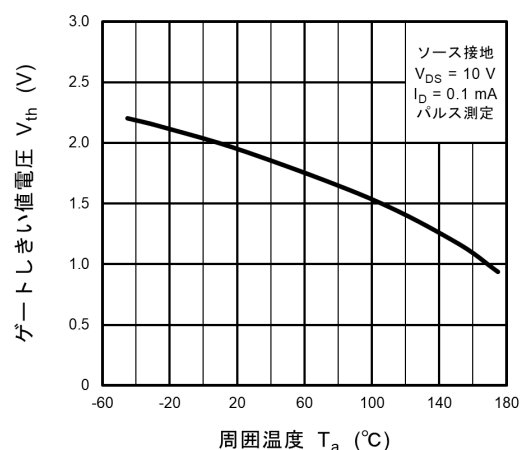
図 9.6 V_{th} - T_a
