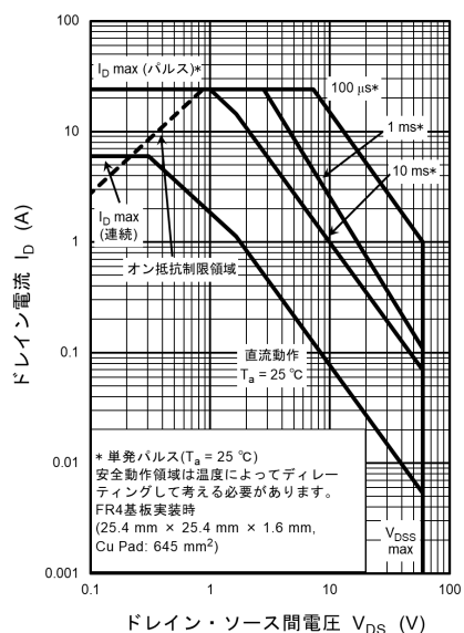
図 9.10 安全動作領域
