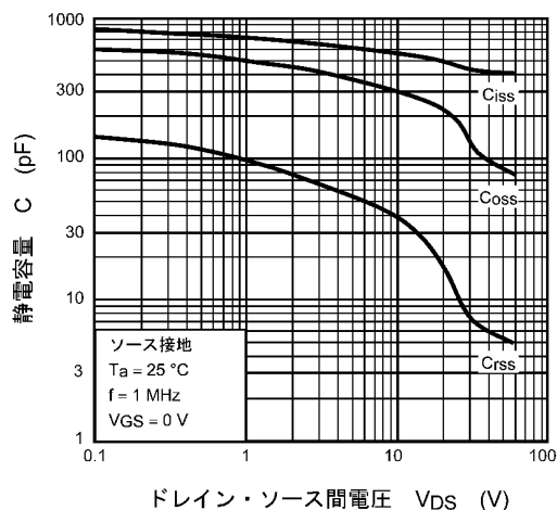
図 9.7 C - V_{DS}
