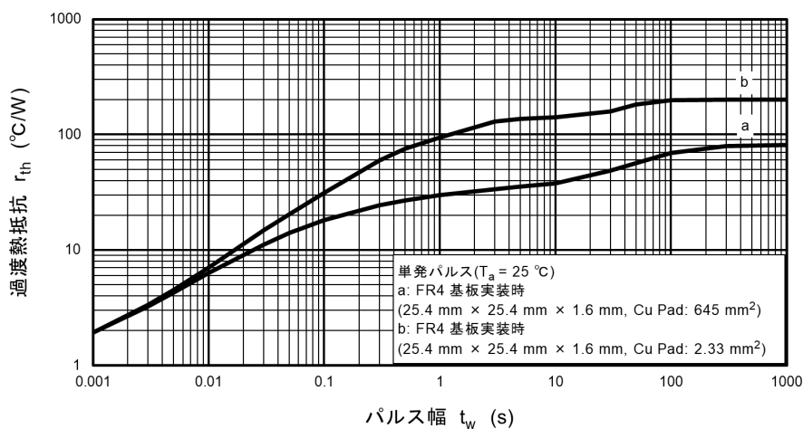
図 9.9 r_{th} - t_w
