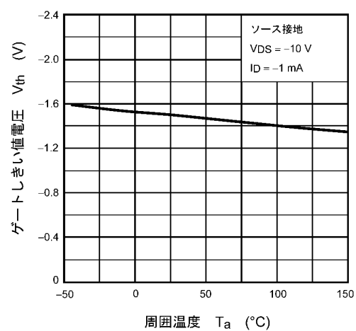
図 9.6 V_{th} - T_a
