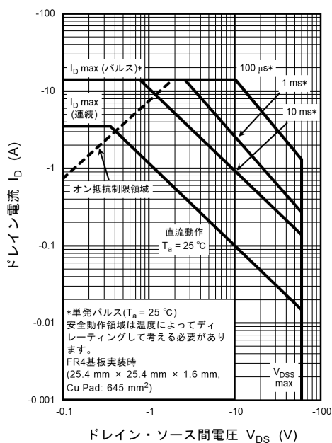
図 9.10 安全動作領域
