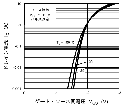
図 9.2 I_D - V_{GS}
