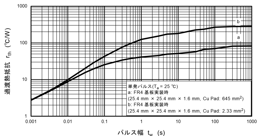
図 9.9 r_{th} - t_w
