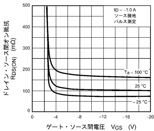
図 9.3 R_{DS(ON)} - V_{GS}
