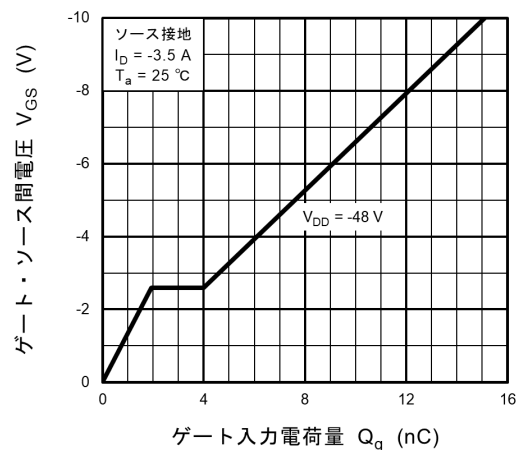
図 9.8 ダイナミック入力特性
