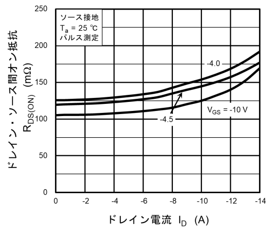
図 9.4 R_{DS(ON)} - I_D
