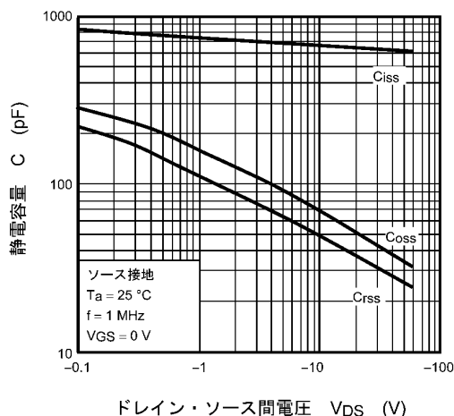
図 9.7 C - V_{DS}
