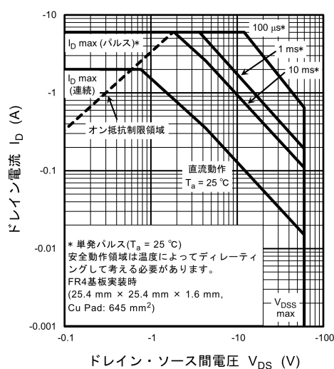
図 9.10 安全動作領域
