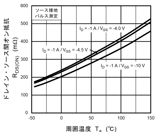
図 9.5 R_{DS(ON)} - T_a
