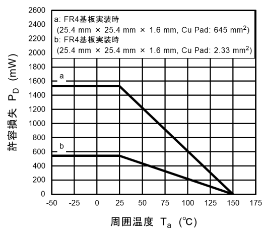
図 9.11 P_D - T_a
