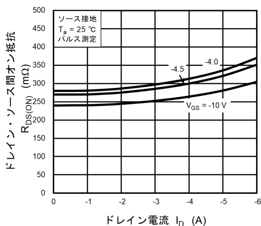
図 9.4 R_{DS(ON)} - I_D
