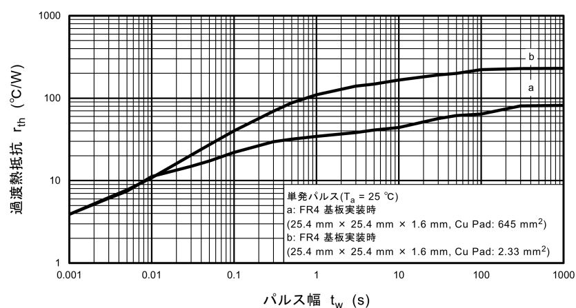
図 9.9 r_{th} - t_w
