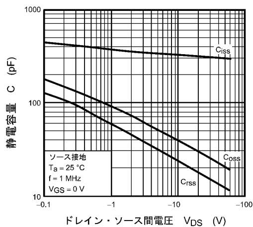
図 9.7 C - V_{DS}
