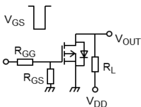
図 6.3.1 スwitchング時間の測定回路
