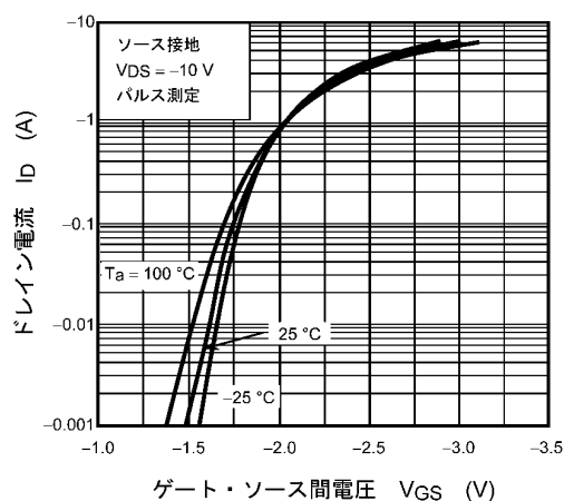
図 9.2 I_D - V_{GS}
