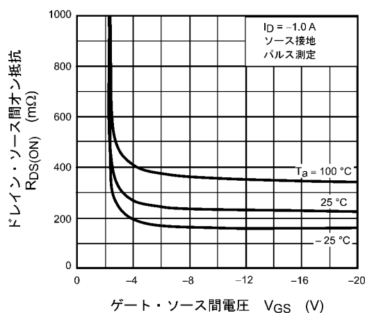
図 9.3 R_{DS(ON)} - V_{GS}
