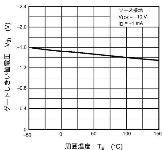
図 9.6 V_{th} - T_a
