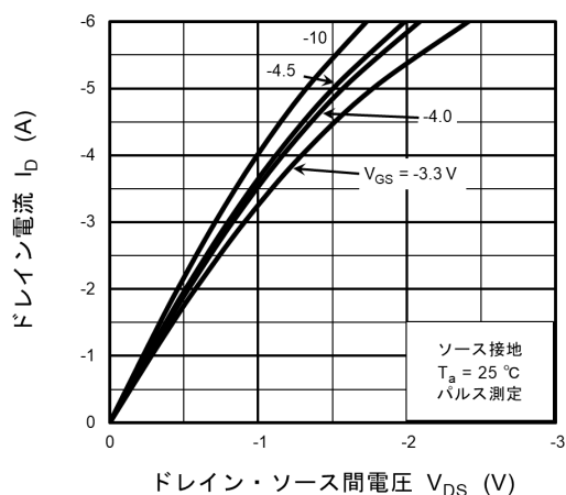
図 9.1 I_D - V_{DS}
