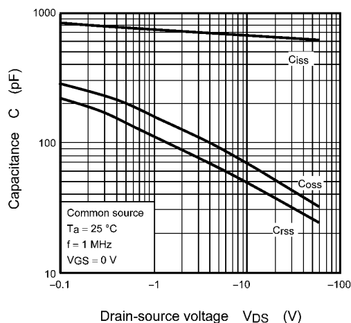
Fig. 9.7 C - V_{DS}
