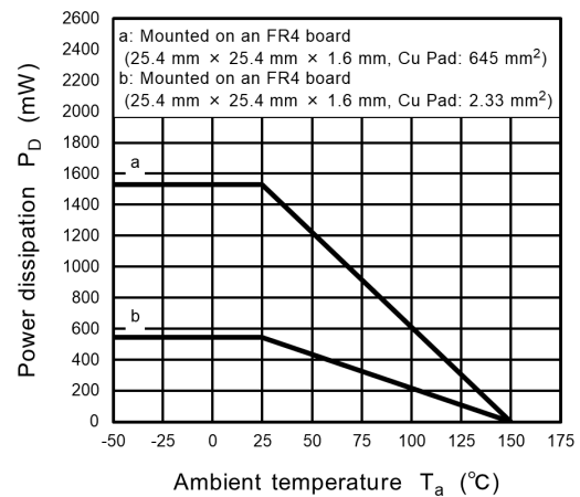
Fig. 9.11 P_D - T_a
