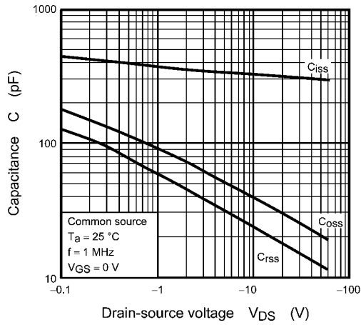
Fig. 9.7 C - V_{DS}
