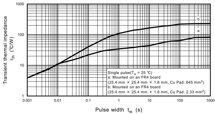
Fig. 9.9 r_{th} - t_w
