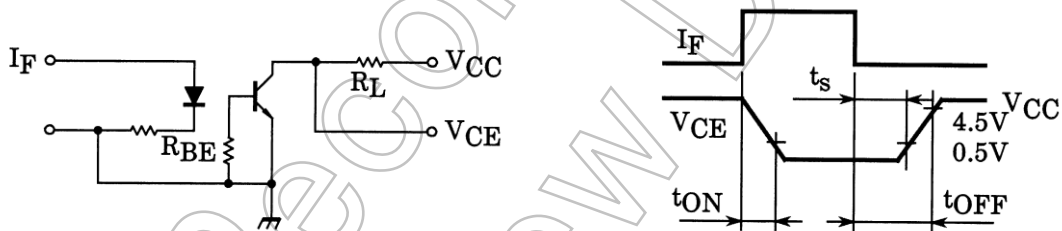
図1: スwitchング時間測定回路
