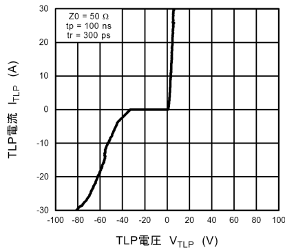
図 10.20.1 I_{TLP} - V_{TLP}
