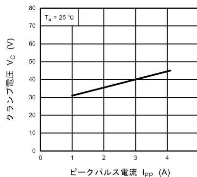
図 10.18.2 V_C - I_{PP}
