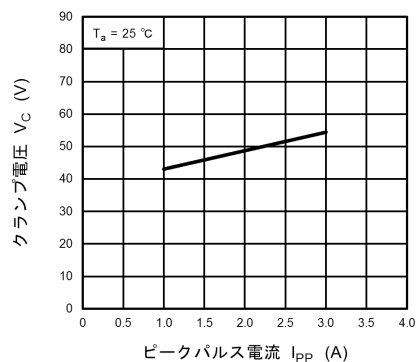
図 10.21.2 V_C - I_{PP}
