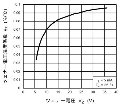
図 10.1.3 \gamma_Z - V_Z
