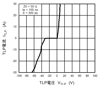
図 10.19.1 I_{TLP} - V_{TLP}
