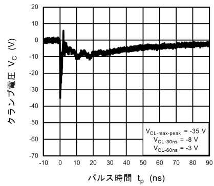
図 10.5.4 IEC61000-4-2 クランプ波形 -8 kV
