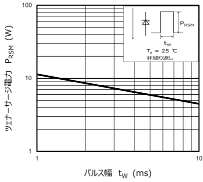
図 10.1.9 P_{RSM} - t_w
