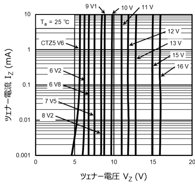
図 10.1.1 I_Z - V_Z(1)
