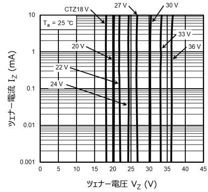
図 10.1.2 I_Z - V_Z(2)
