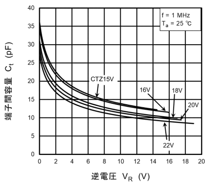
図 10.1.7 C_t - V_R(3)
