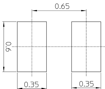
図 9.1 参考パッド寸法(Unit: mm)
