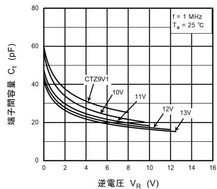
図 10.1.6 C_t - V_R(2)
