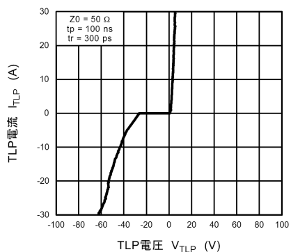
図 10.18.1 I_{TLP} - V_{TLP}
