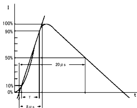
図 10.22.1 V_C - I_{PP} 印加波形 (IEC61000-4-2準拠 8/20 \mu s pulse)
