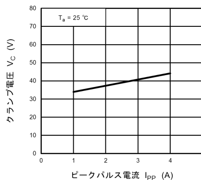
図 10.19.2 V_C - I_{PP}
