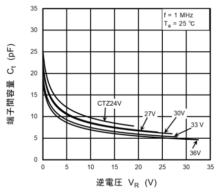
図 10.1.8 C_t - V_R(4)
