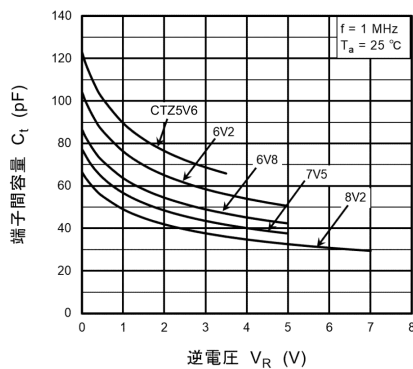
図 10.1.5 C_t - V_R(1)
