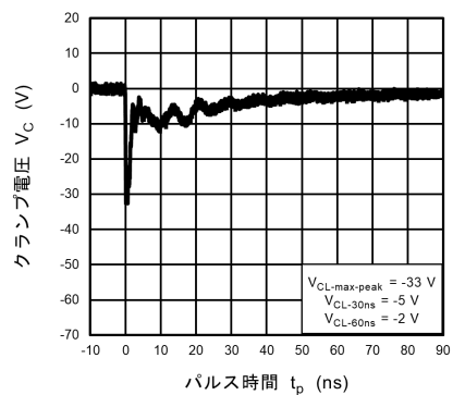
図 10.21.4 IEC61000-4-2 クランプ波形 -8 kV
