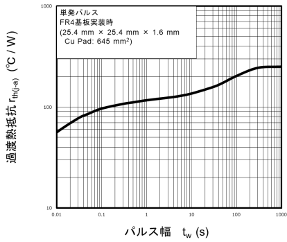
図 10.1.11 r_{th(j-a)} - t_w
