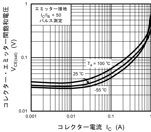
図 7.1.3 V_{CE(sat)} - I_C
