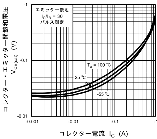
図 7.2.3 V_{CE(sat)} - I_C
