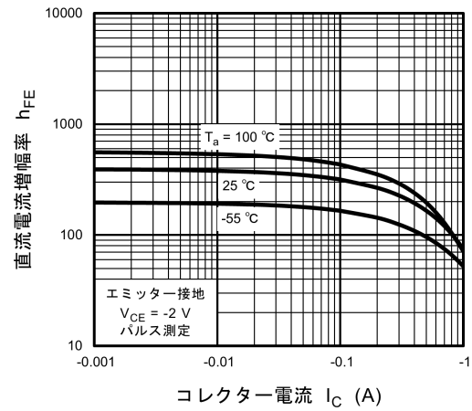
図 7.2.2 h_{FE} - I_C
