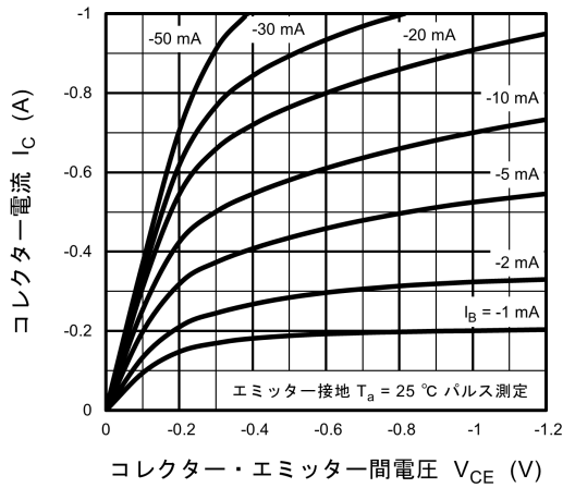
図 7.2.1 I_C - V_{CE}
