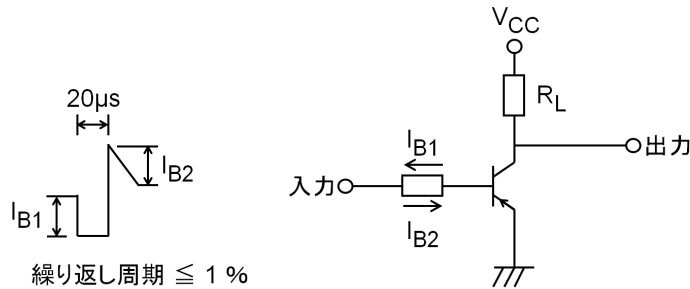
図 5.4.1 スwitching時間の測定回路
