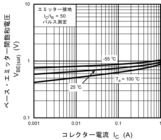
図 7.1.4 V_{BE(sat)} - I_C
