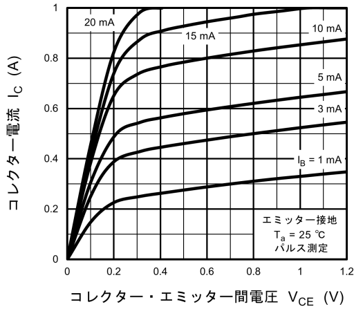
図 7.1.1 I_C - V_{CE}
