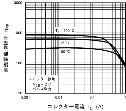
図 7.1.2 h_{FE} - I_C
