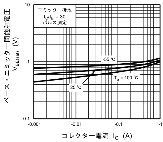
図 7.2.4 V_{BE(sat)} - I_C
