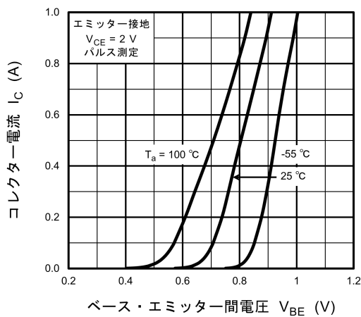
図 7.1.5 I_C - V_{BE}
