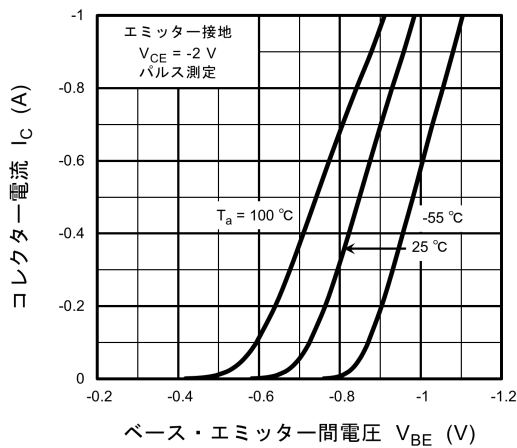
図 7.2.5 I_C - V_{BE}
