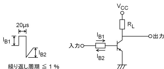
図 5.2.1 スwitchング時間の測定回路
