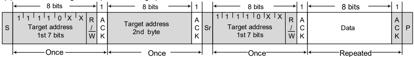
(d) 10-bit addressing format (read from target)
