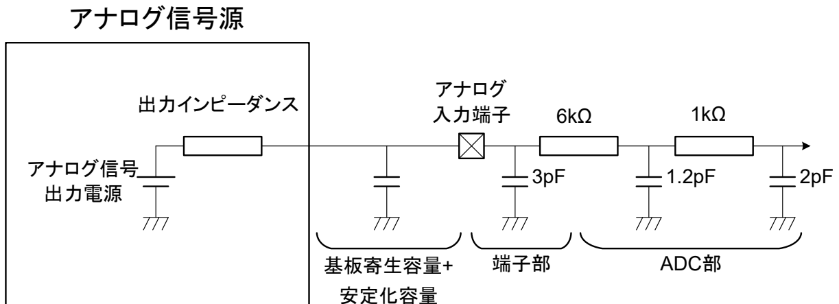
図 3.5 アナログ入力等価回路
