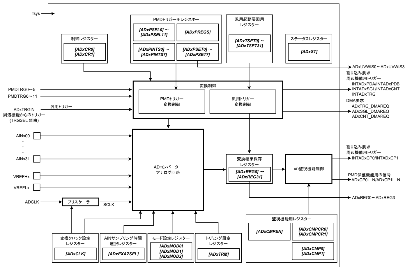
図 2.1 ADCブロック図
