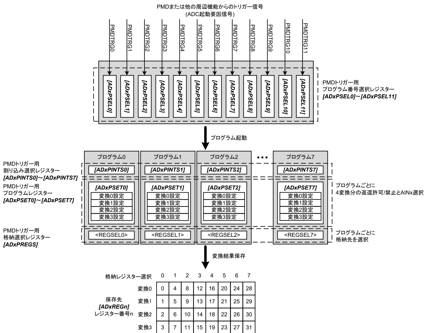
図 3.2 PMDトリガー起動と関連レジスター
