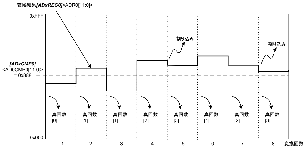
図 3.4 AD監視機能(判定カウント累積方式)
