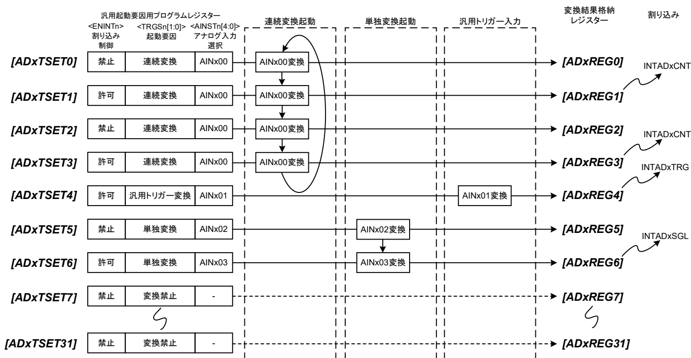
図 3.1 汎用起動要因の変換動作
