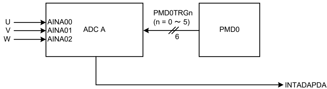
図 5.1 3シャントの例
