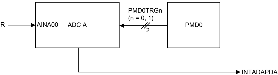
図 5.2 1 シャントの例
