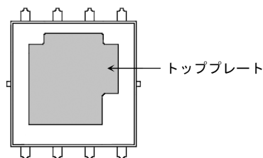
図 5.3 上面図
