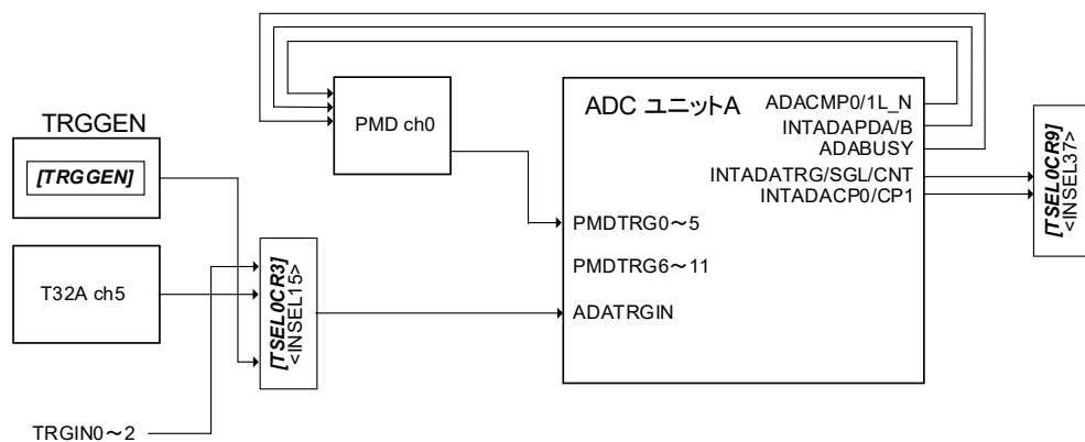
図 2.2 ADCと周辺機能の接続
