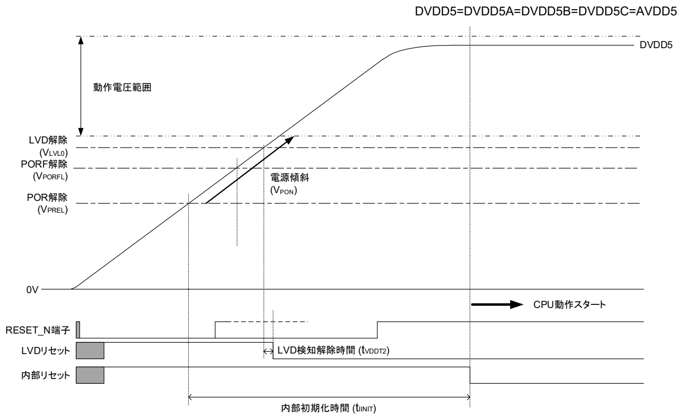
図 3.3 RESET_N端子によるリセット動作(2)
