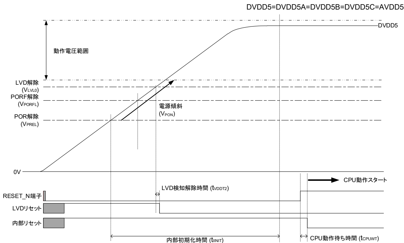
図 3.2 RESET_N端子によるリセット動作(1)
