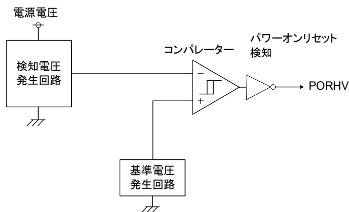
図 3.8 パワーオンリセット回路
