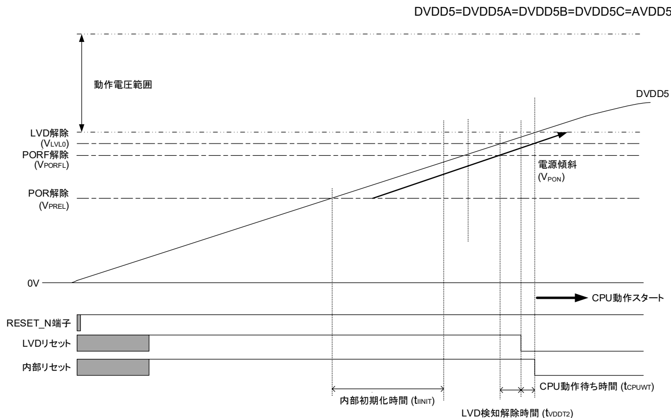
図 3.4 LVDリセットによるリセット動作
