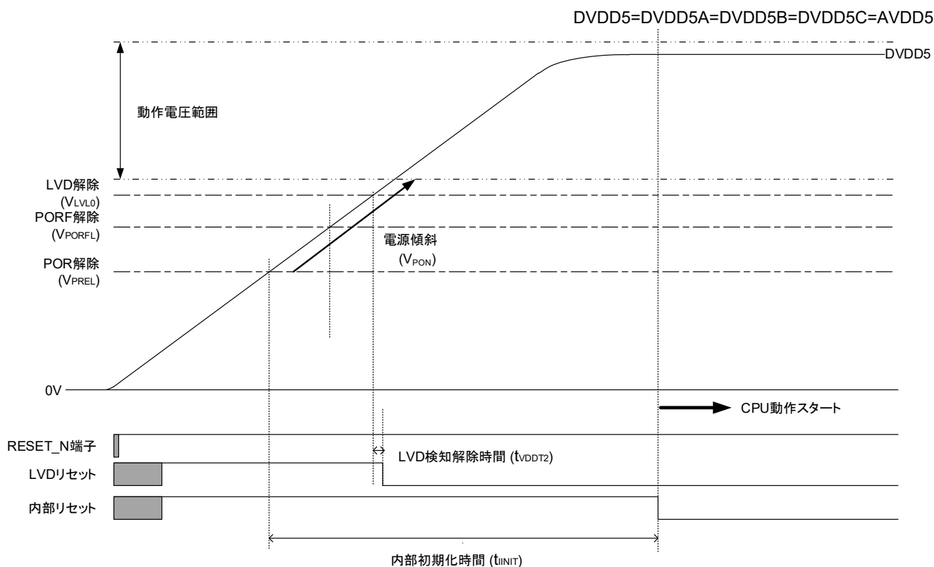
図 3.1 パワーオンリセット回路によるリセット動作
