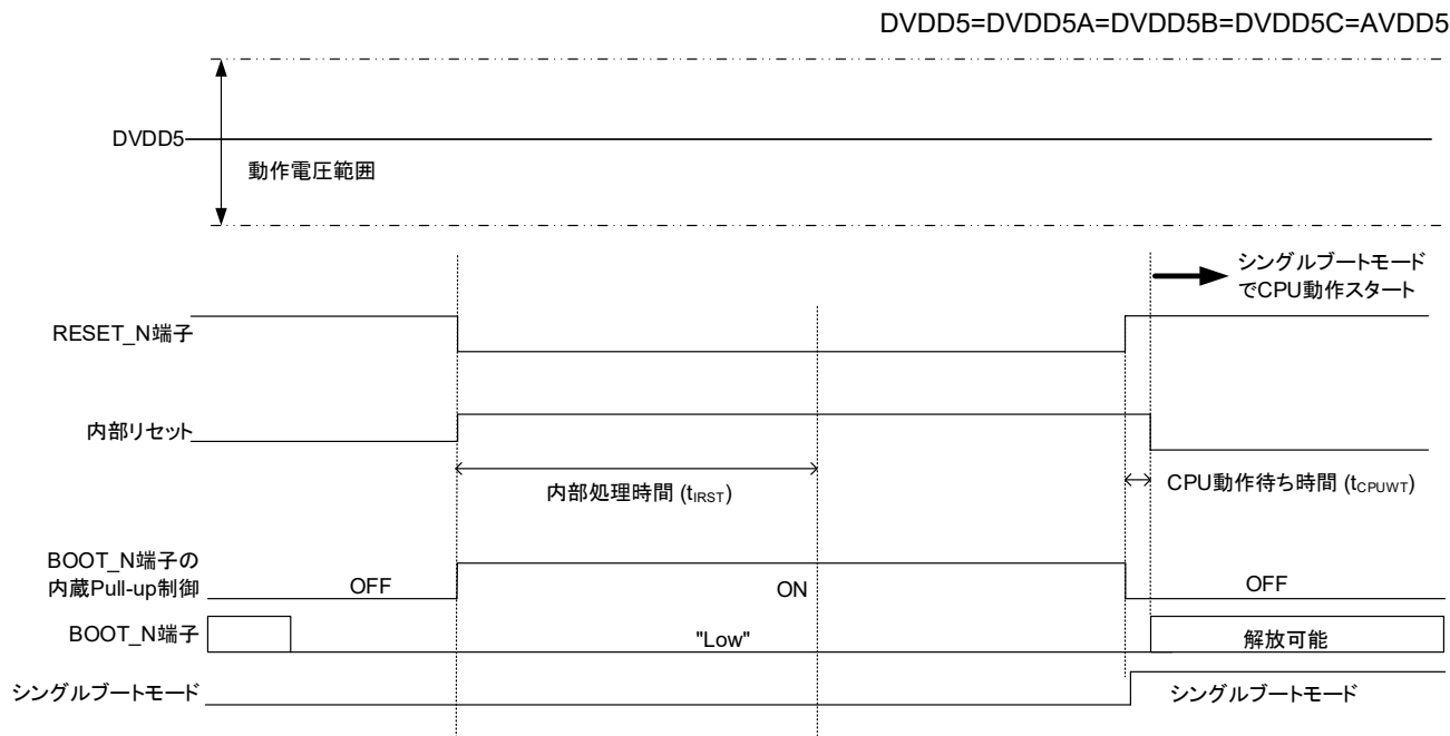
図 3.7 電源安定時のシングルブートモードの起動
