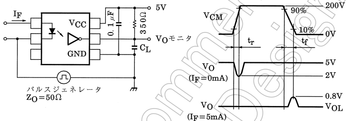
図2 コモンモードノイズ測定回路、波形
