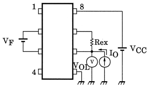
図 5 VoL 測定回路
