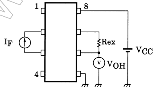
図 4 V_{OH} 測定回路
