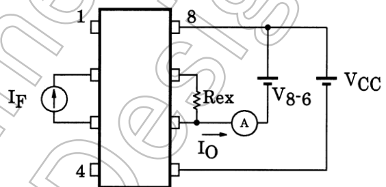
図 3 I_O 測定回路
