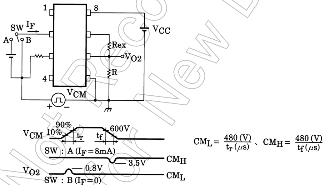
図 7 CM_H 、 CM_L 測定回路
