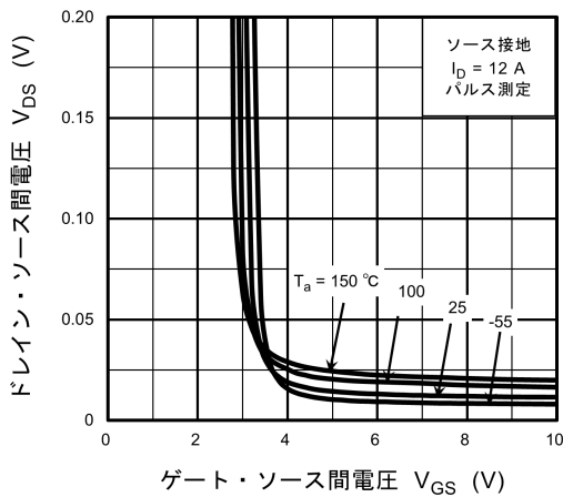
図 8.5 V_{DS} - V_{GS}
