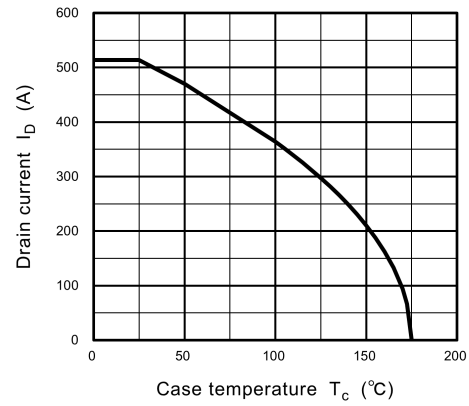
Fig. 8.15 I_D - T_c
