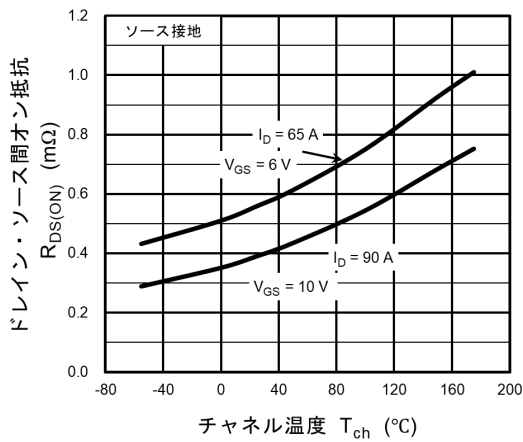
図 8.9 R_{DS(ON)} - T_a
