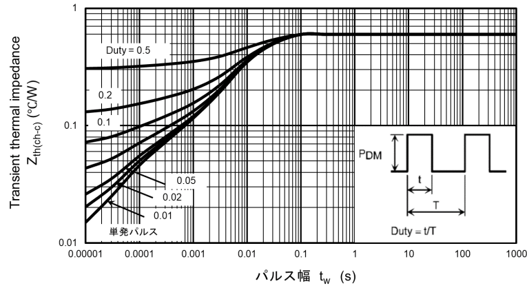
図 8.13 r_{th} - t_w (最大値 (保証値))
