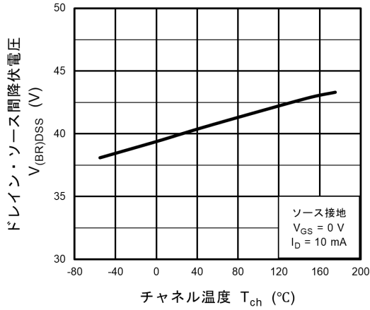
図 8.7 V_{(BR)DSS} - T_a
