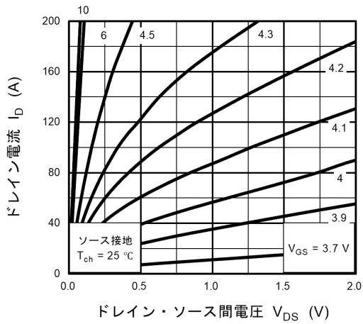
図 8.1 I_D - V_{DS}
