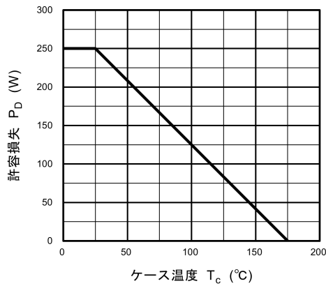
図 8.14 P_D - T_c (最大値 (保証値))
