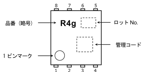
図 7.1 現品表示
