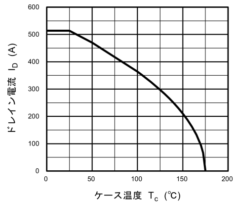
図 8.15 I_D - T_c
