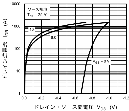
図 8.5 I_{DR} - V_{DS}
