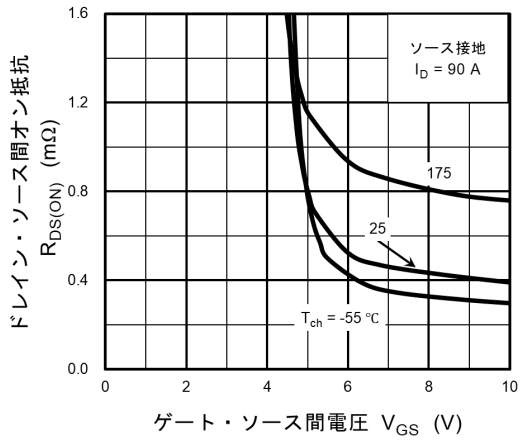
図 8.3 R_{DS(ON)} - V_{GS}
