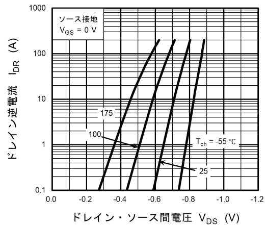
図 8.6 I_{DR} - V_{DS}
