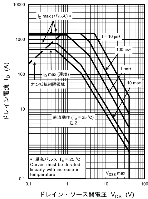
図 8.16 安全動作領域 (最大値 (保証値))
