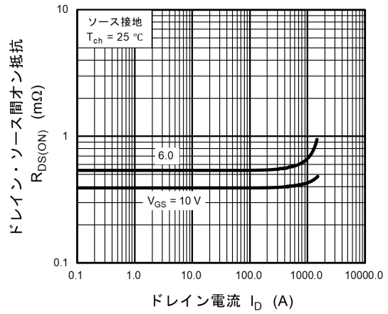
図 8.4 R_{DS(ON)} - I_D
