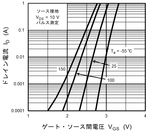
図 8.7 I_D - V_{GS}
