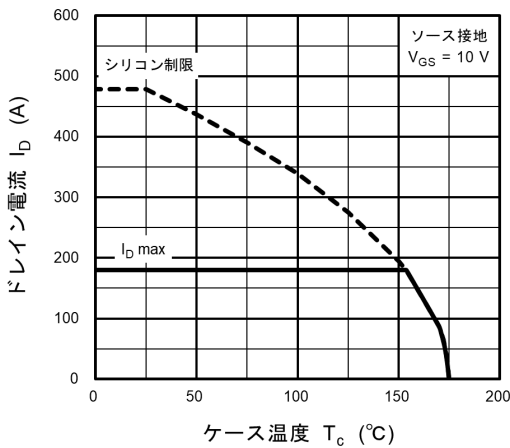
図 8.18 I_D - T_c
