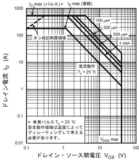
図 8.16 安全動作領域 (最大値 (保証値))
