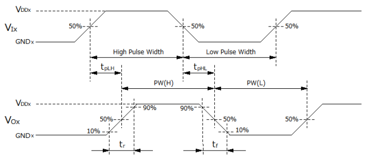
図 12-1-4: DCL34xx0B Switching 特性波形図
