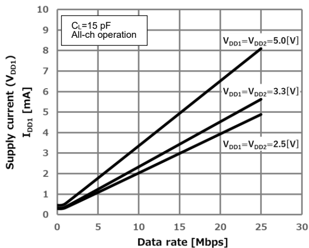
図 13.5. DCL342x0B I_{DD1} 動作電流—データレート
