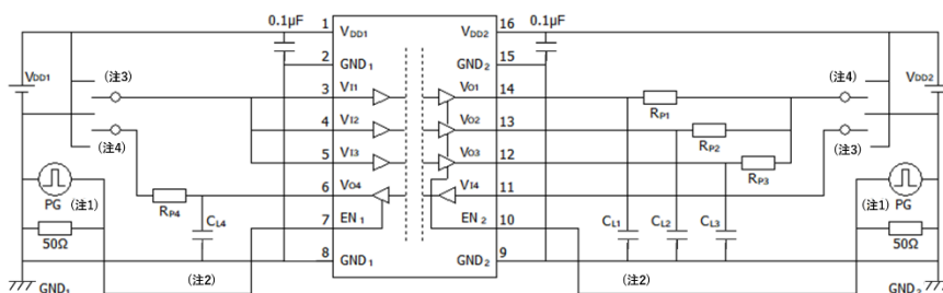
図 12-2-2: DCL341L0B/DCL341H0B イネーブル伝搬遅延時間テスト回路図
