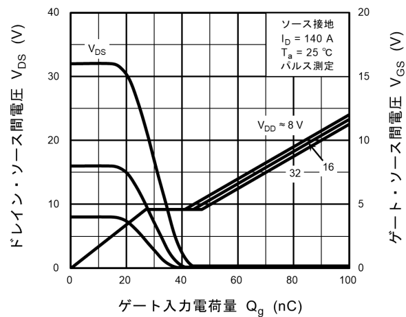
図 8.14 ダイナミック入出力特性
