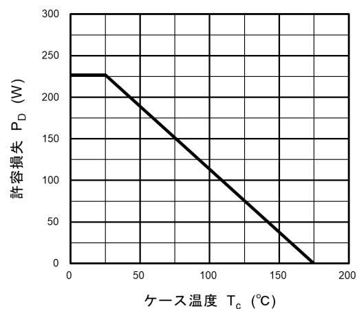
図 8.17 P_D - T_c (最大値 (保証値))
