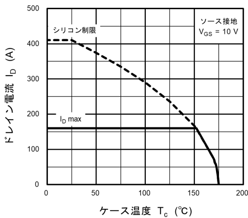
図 8.18 I_D - T_c
