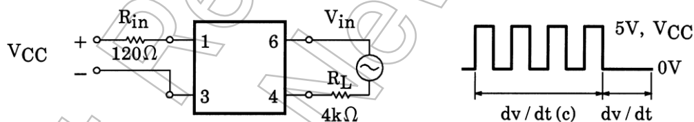
図 1: dv/dt 測定回路
