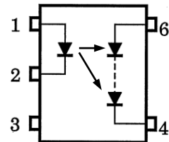
ピン接続図(Top View)
