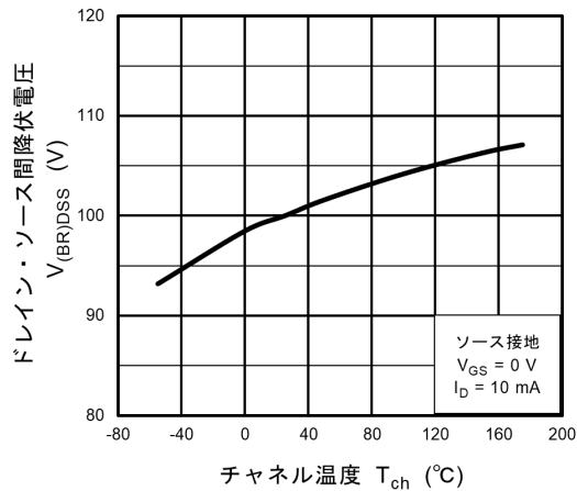
図 8.7 V_{(BR)DSS} - T_{ch}
