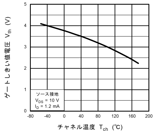
図 8.8 V_{th} - T_{ch}
