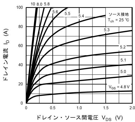
図 8.1 I_D - V_{DS}
