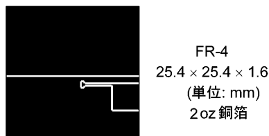
図 5.1 ガラスエポキシ基板 実装例
