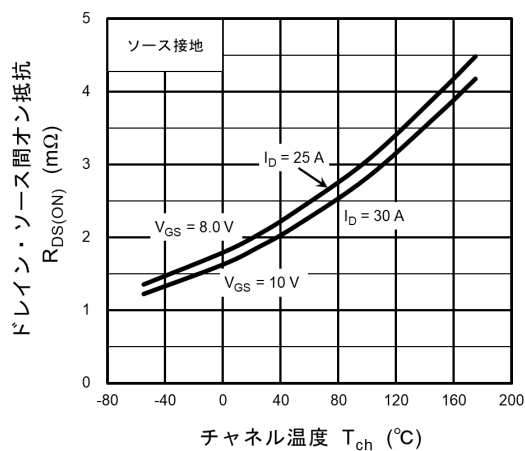
図 8.9 R_{DS(ON)} - T_{ch}
