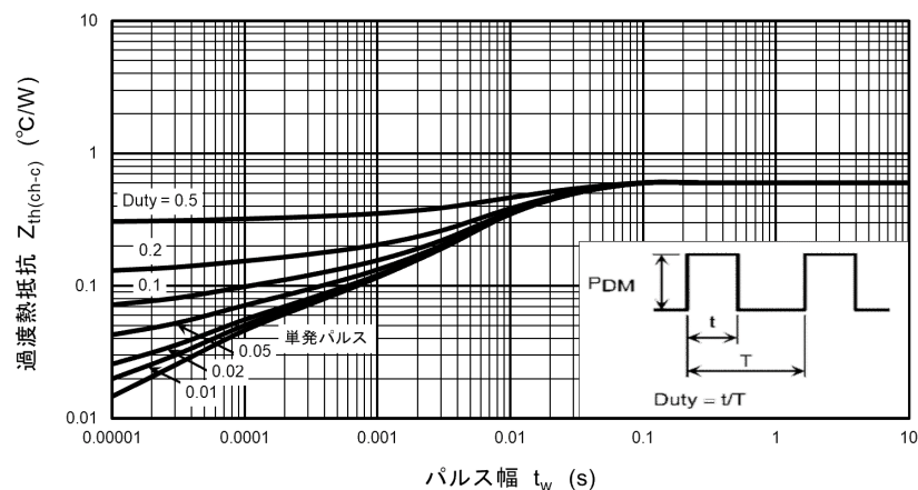
図 8.13 Z_{th(ch-c)} - t_w (最大値 (保証値))
