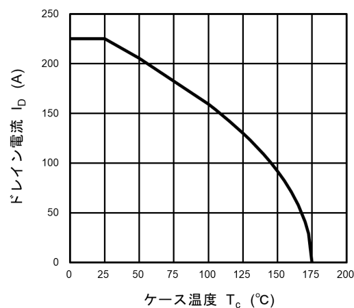
図 8.15 I_D - T_c
