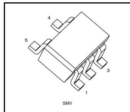
SMV (SOT-25) (SC-74A) 質量: 16 mg (標準)
