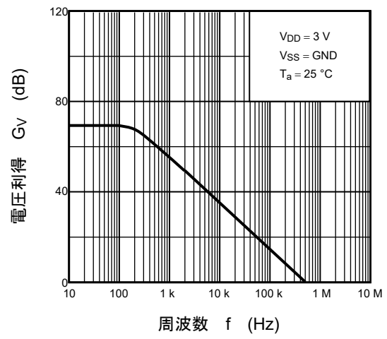
図 7.2 G_V - f
