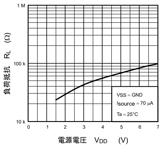
図 7.3 R_L - V_{DD}
