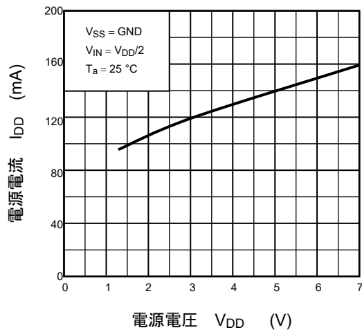
図 7.1 I_{DD} - V_{DD}
