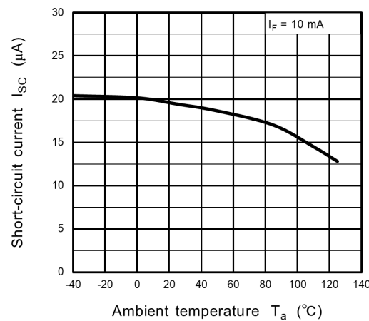
Fig. 11.6 I_{SC} - T_a
