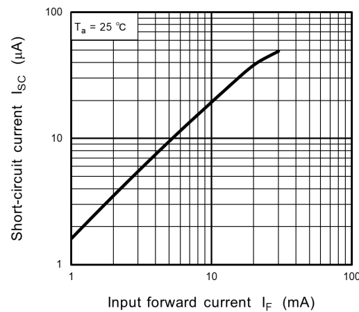
Fig. 11.4 I_{SC} - I_F
