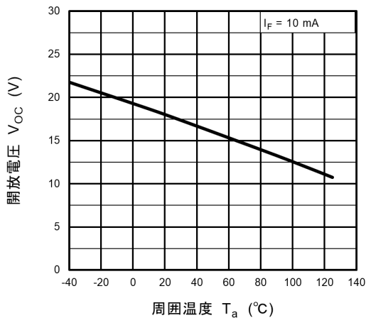
図 11.5 V_{OC} - T_a
