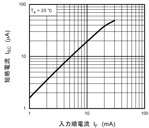
図 11.4 I_{SC} - I_F
