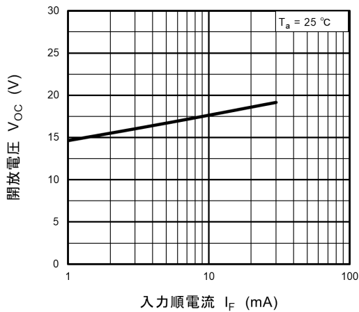
図 11.3 V_{OC} - I_F
