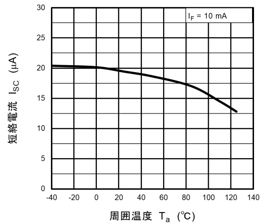
図 11.6 I_{SC} - T_a
