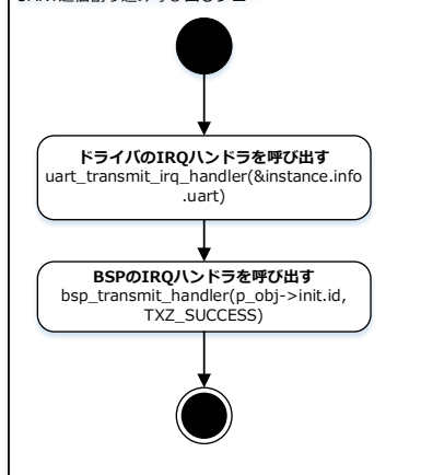
UART送信割り込み呼び出しフロー
