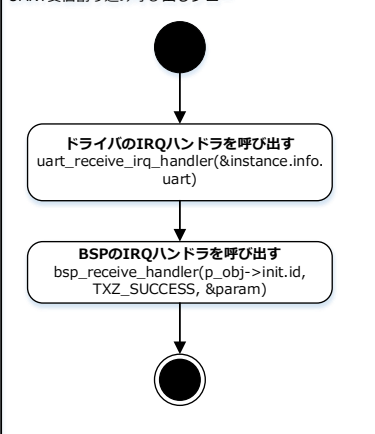
UART受信割り込み呼び出しフロー
