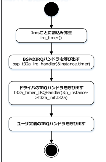
1msタイマー割り込み呼び出しフロー
