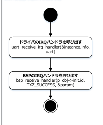
UART受信割り込み呼び出しフロー
