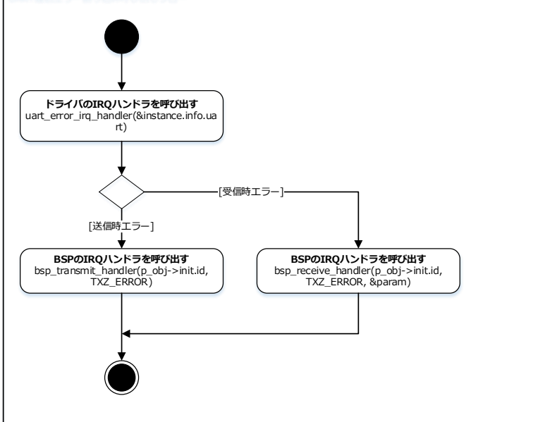
UART通信エラー割り込み呼び出しフロー
