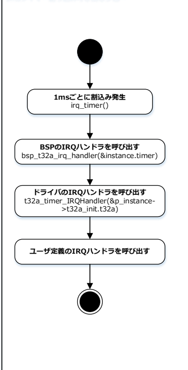
1msタイマー割り込み呼び出しフロー
