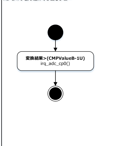
AD CMP0 割り込み呼び出しフロー
