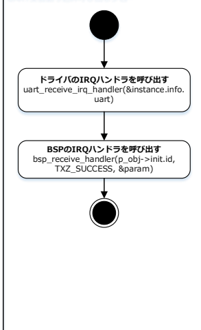
UART受信割り込み呼び出しフロー
