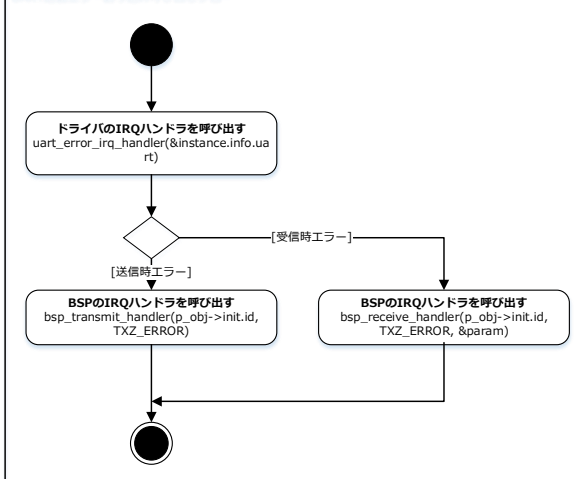
UART送信エラー割り込み呼び出しフロー
