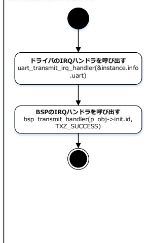
UART送信割り込み呼び出しフロー
