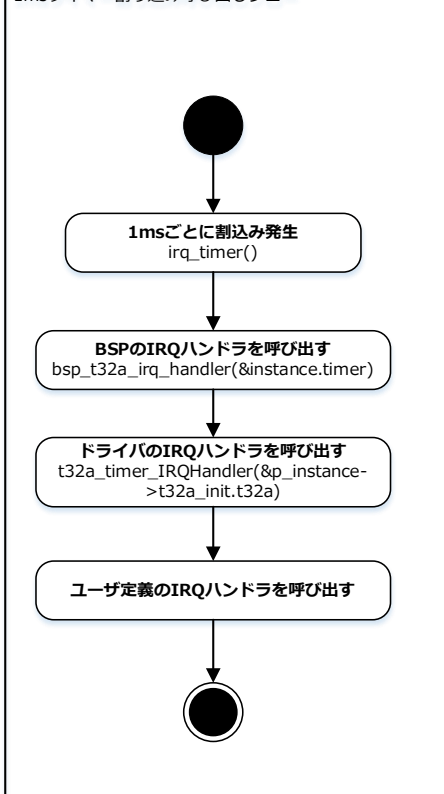
1msタイマー割り込み呼び出しフロー
