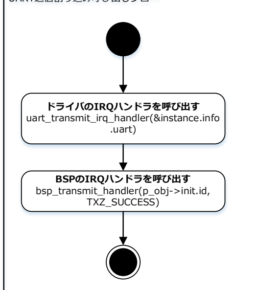
UART送信割り込み呼び出しフロー
