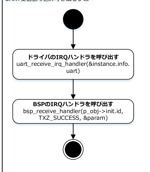
UART受信割り込み呼び出しフロー
