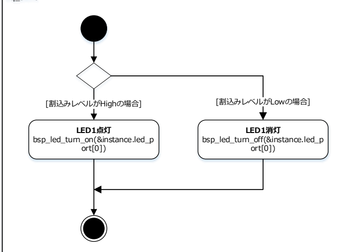
irq_exint
